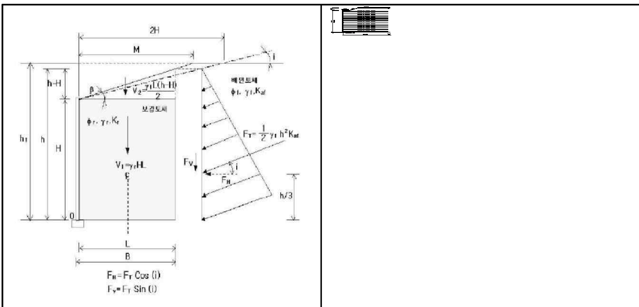
【그림 74.11】 검토단면도
