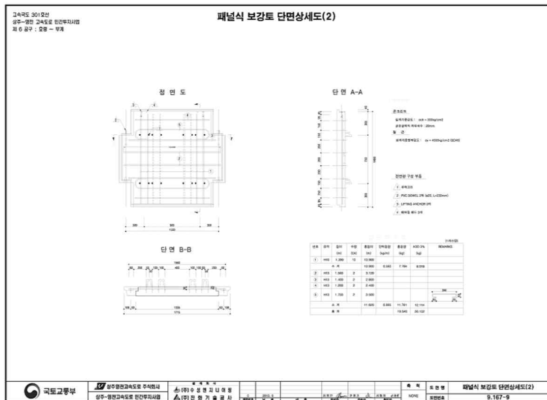
【그림 8.5】 단면도(계속)
