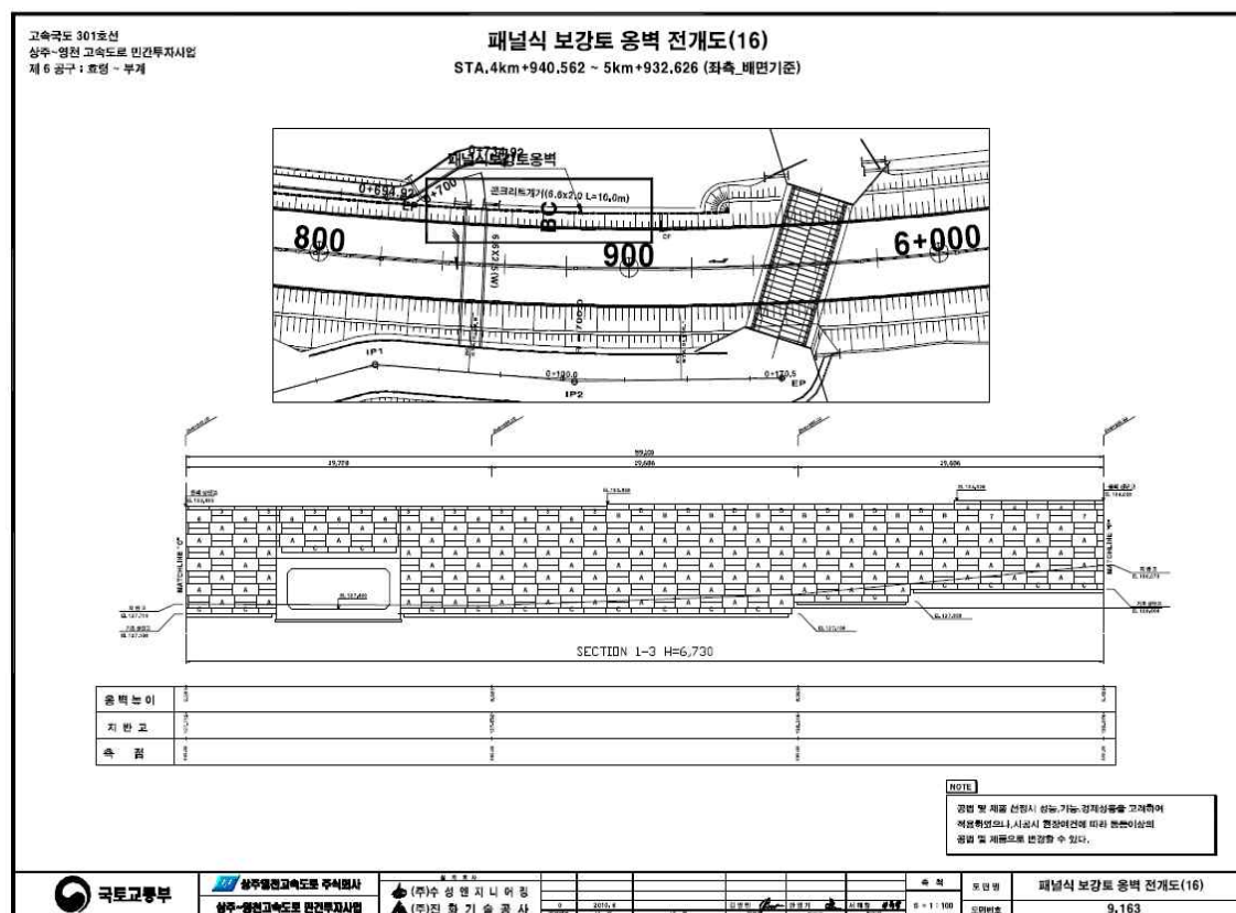
【그림 8.4】 전개도(계속)
