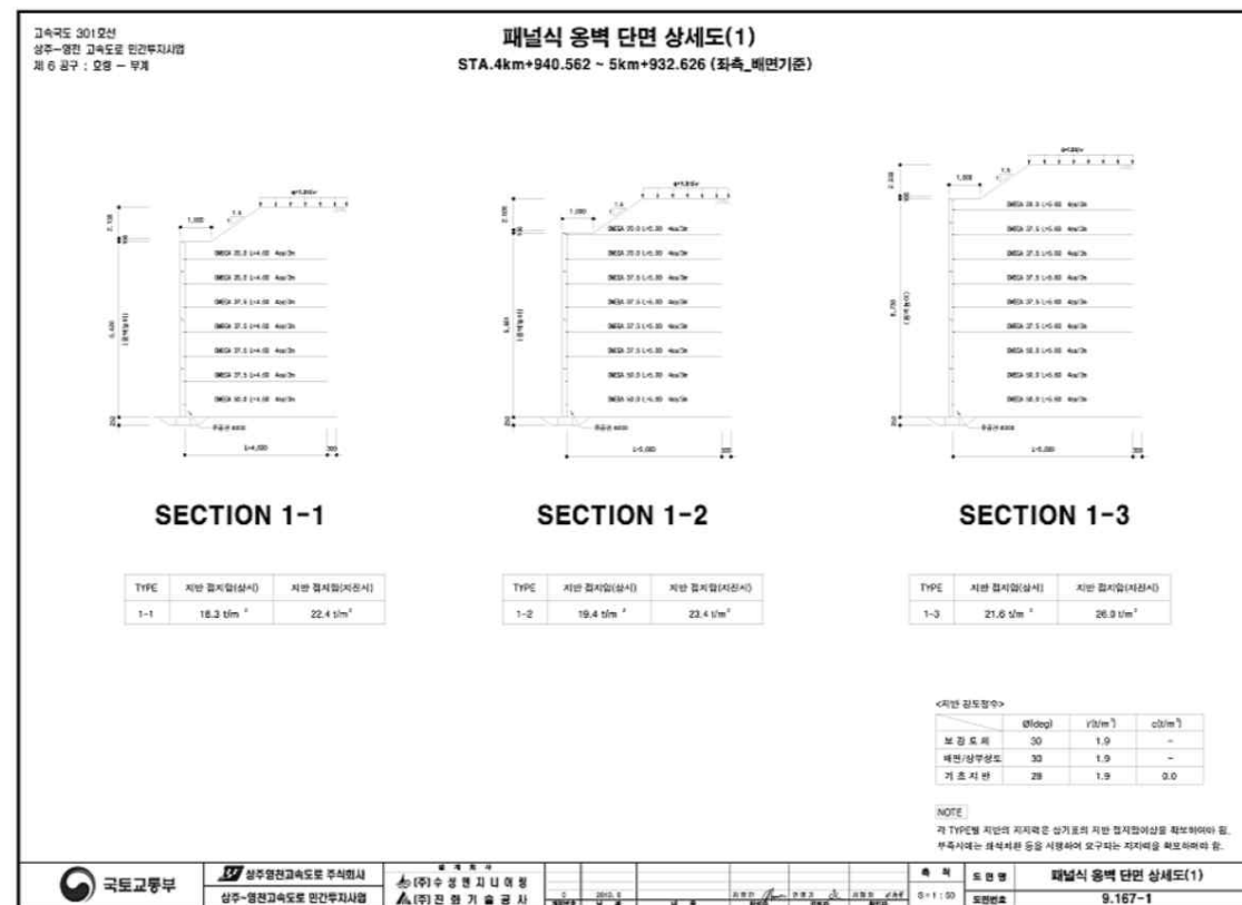
【그림 74.5】 단면도
