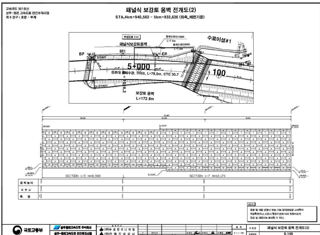
【그림 74.4】전개도
