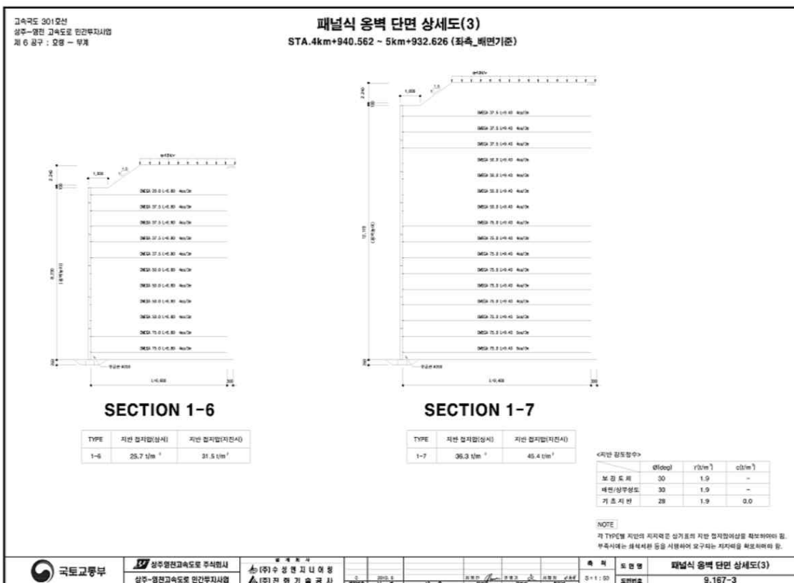
【그림 8.5】 단면도(계속)
